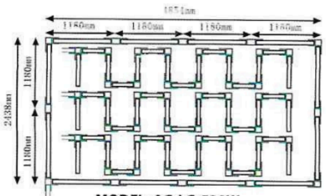
MODEL: AG-LG-520W
